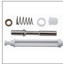
PRO-471-K Воздушный клапан в сборе для PRI Pro Lite
