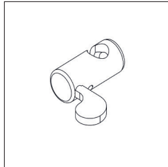
SPA-424-K Зажимной кулачок для AG-362 – поз. № 32
