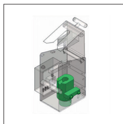
240-3198-L Держатель Ransburg RansFlex для камеры для промывки краскораспылителей 240-3119-1
